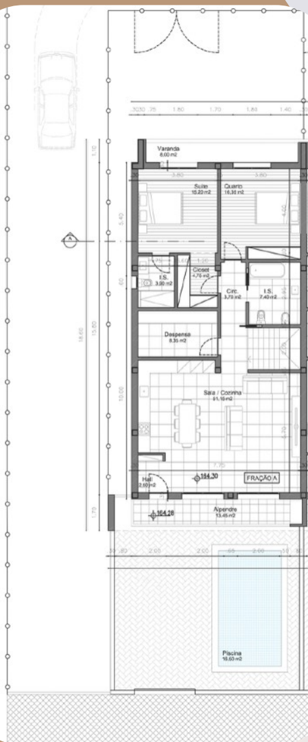
Planta Piso R/C
